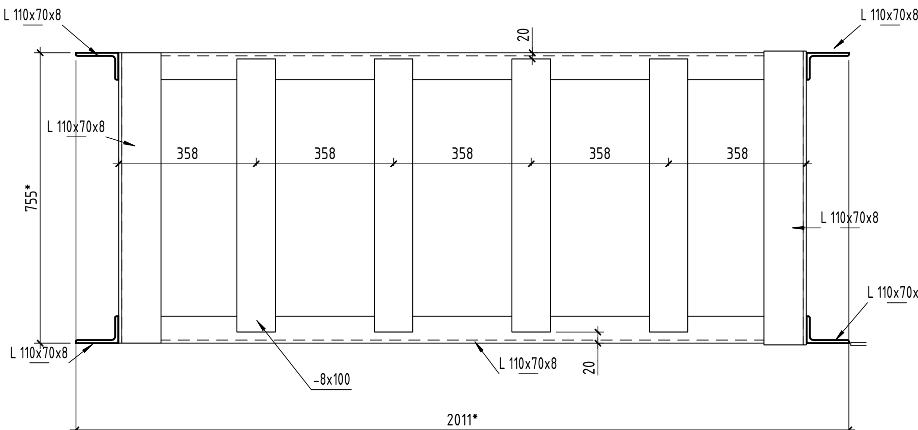
Разрез 1-1 ( 1 : 10
