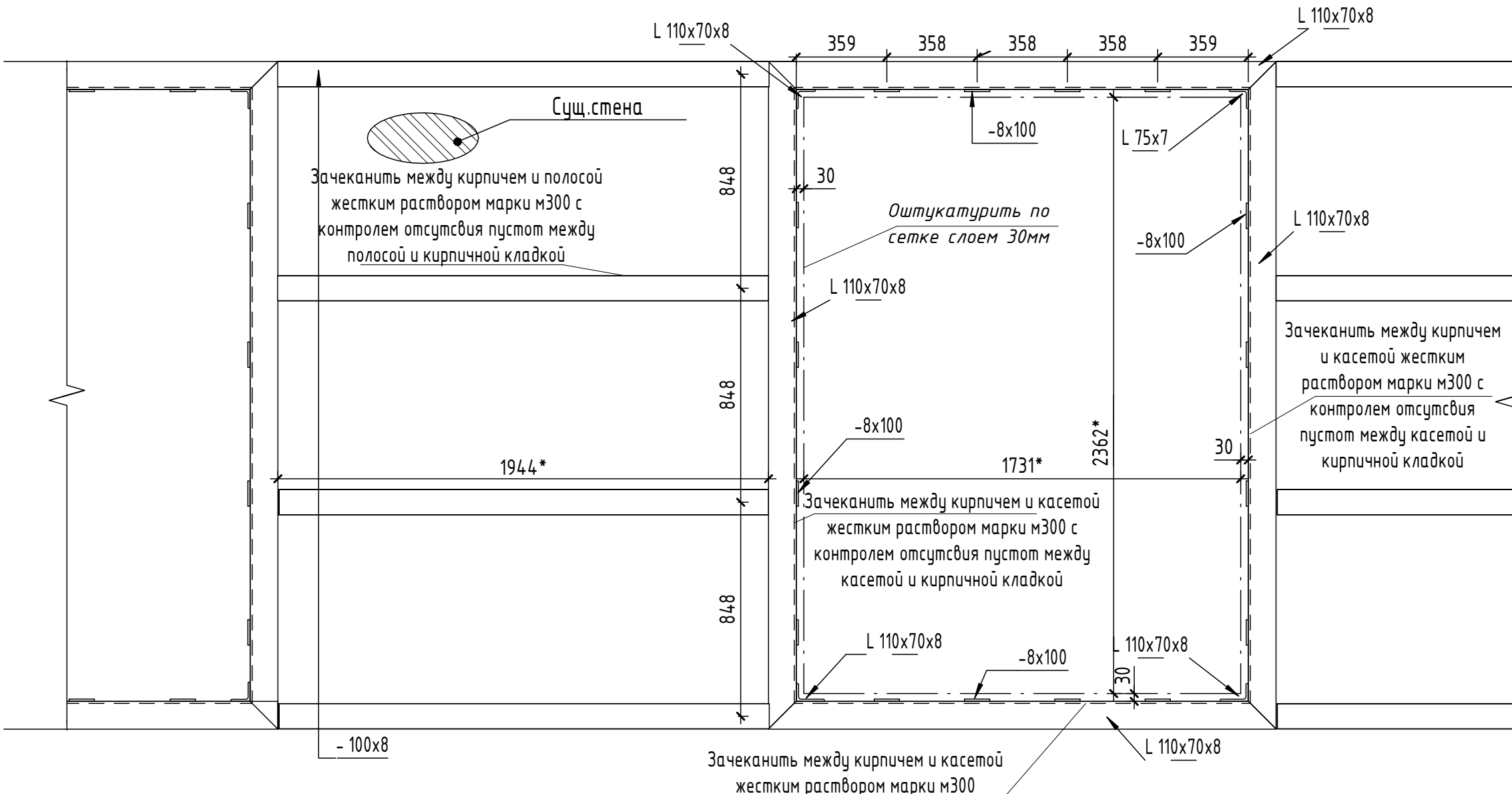
Разрез 1-1 ( 1 : 10
