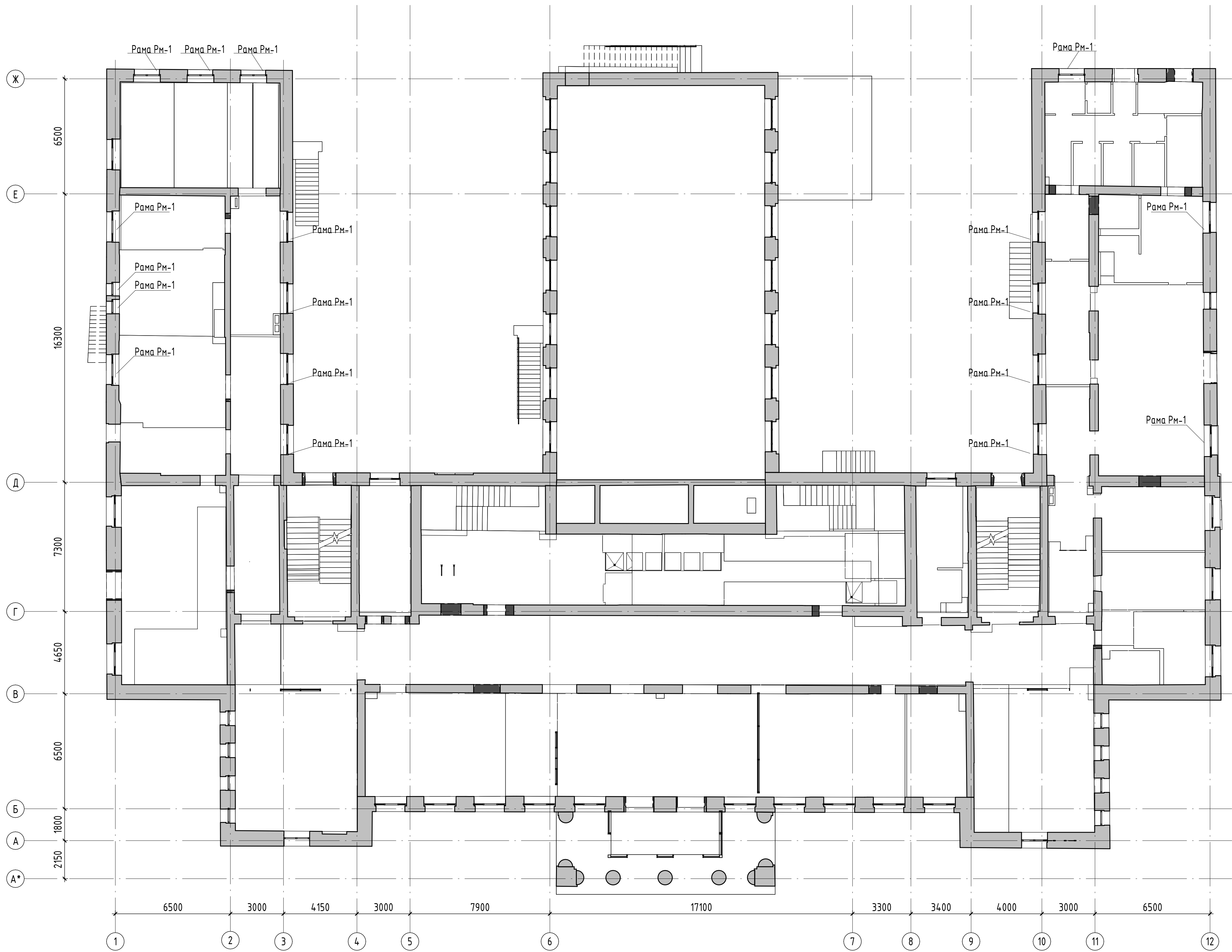
Маркировочный план рам усиление оконных проемов 1 этажа в осях 1-3/Д-Ж и 10-12/Д-Ж (1 : 100)
