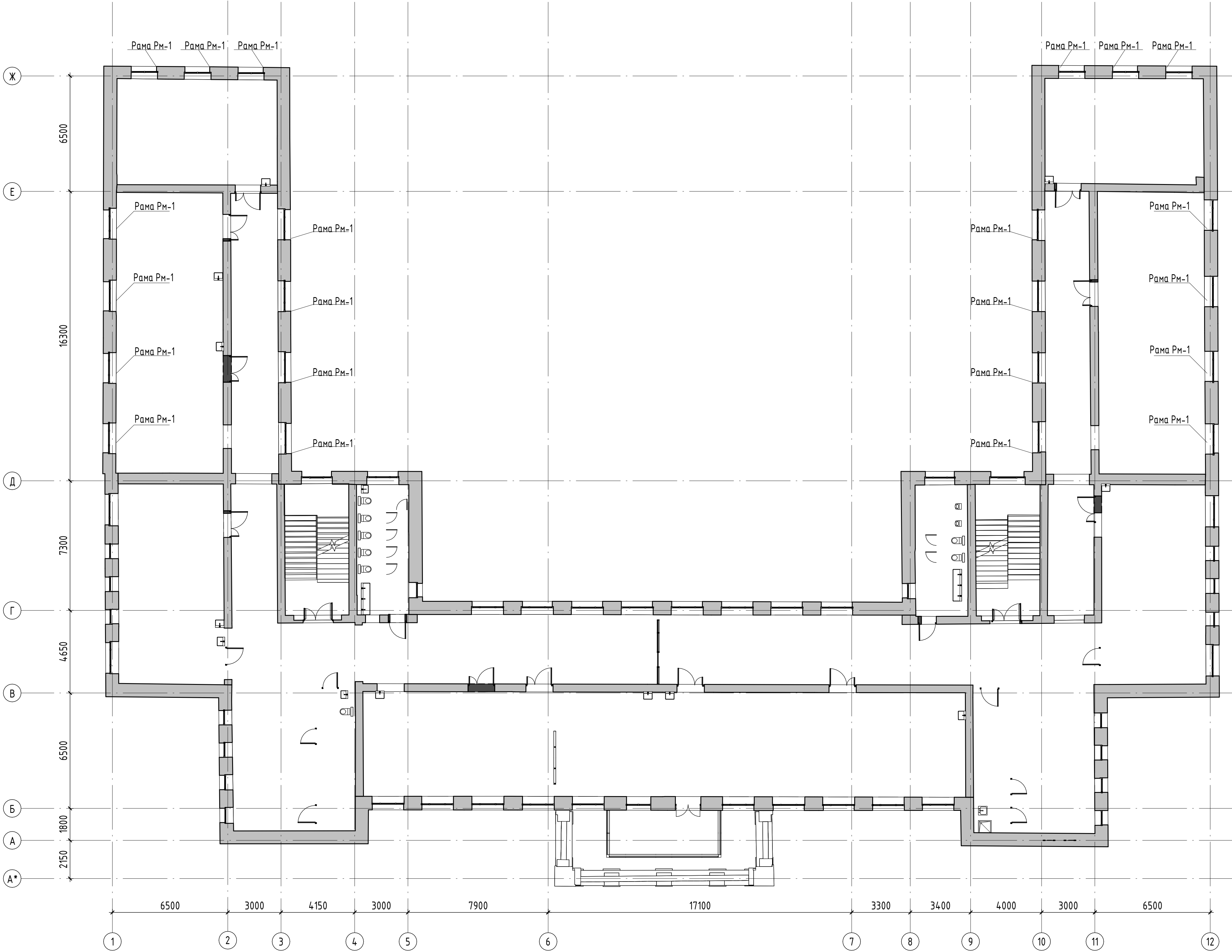
Маркировочный план рам усиление оконных проемов 2 этажа в осях 1-3/Д-Ж и 10-12/Д-Ж (1 : 100)
